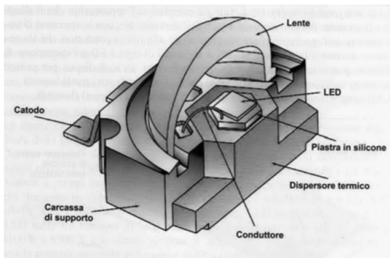
Figura 9: Componenti del LED
