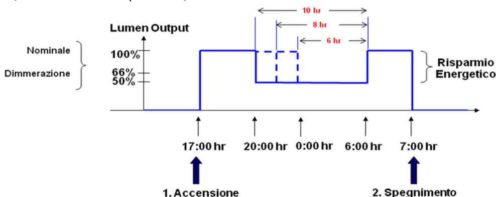
Figura 11: Sistema di dimmerazione
