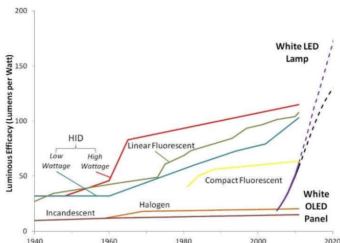
Figura 10: Andamento dell'efficienza dei diversi tipi di lampade negli ultimi anni
