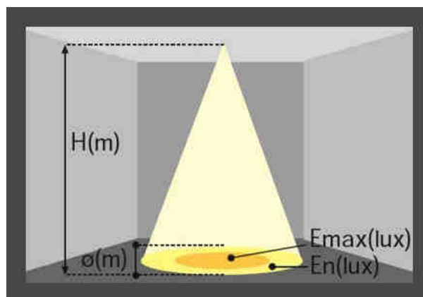
Figura 7: Esempio di illuminamento di un punto luce
