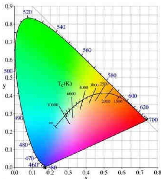
Figura 5: Diagramma cromatico con curva di Plank
