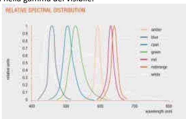
Figura 8: Distribuzione spettrale dei LED
