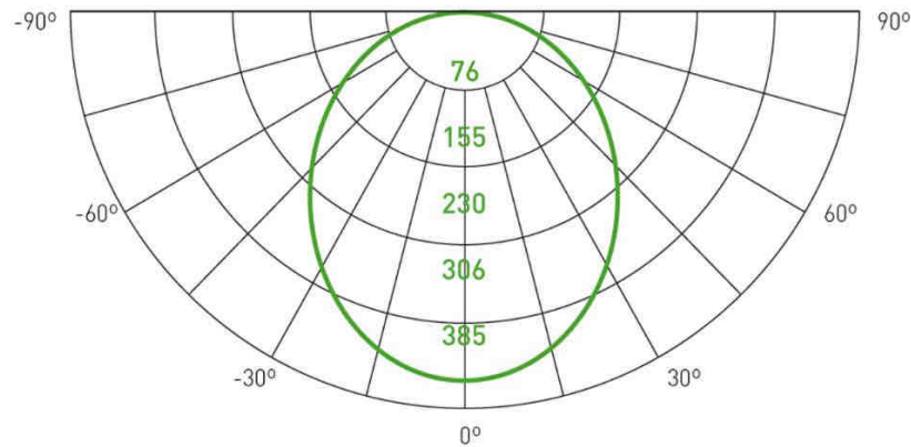
Figura 6: Esempio di curva fotometrica
